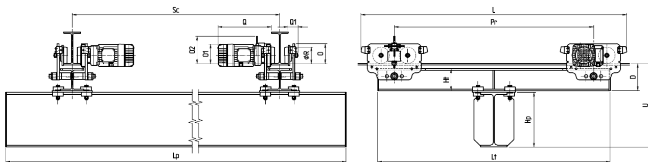
Ponte sospeso DPS1 – Portata 1000 kg – Paranco DRH1
