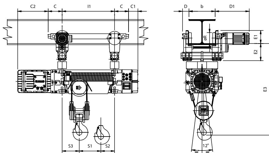
Configuration avec chariot avec bride oscillant O
