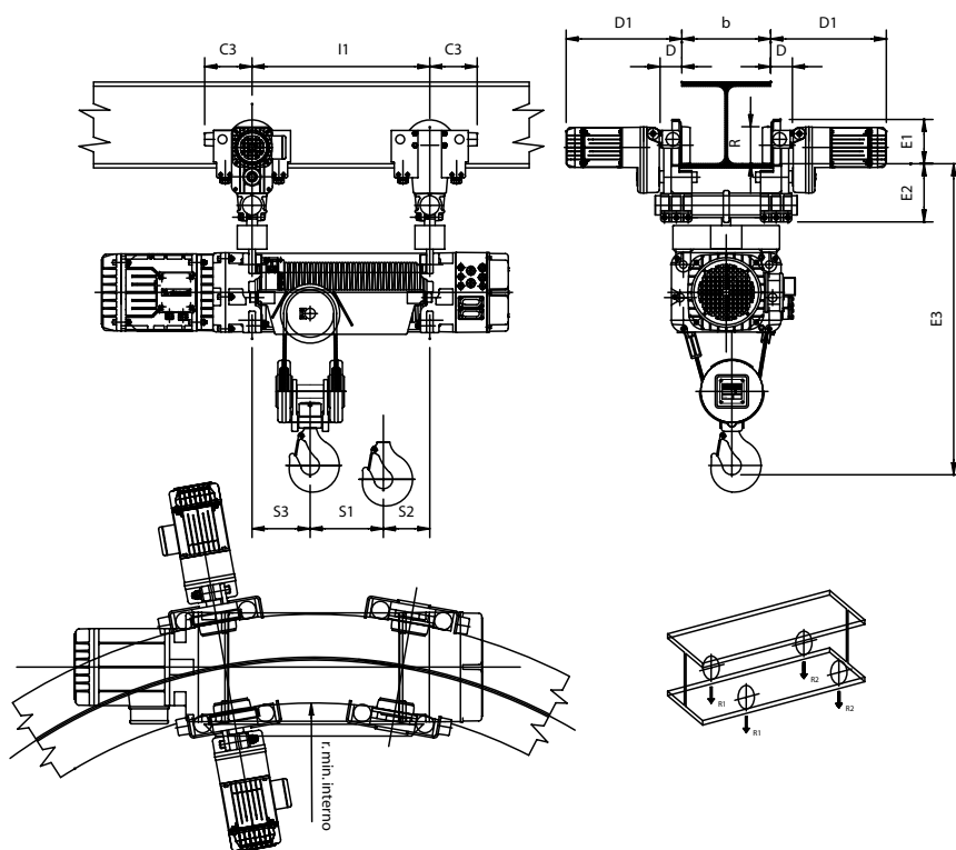
Configuration avec chariot articulé S
