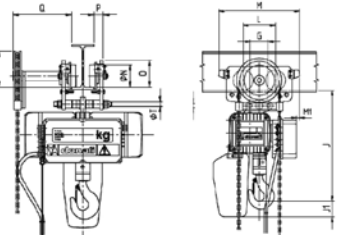
Polipasto con carro de cadena CM
