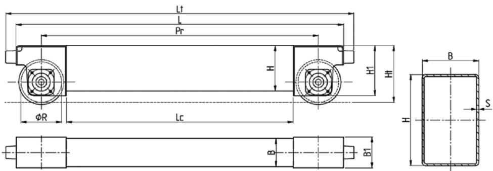
Gesamtbild Laufkatze
