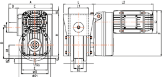
Antriebs-Laufvorrichtungen
