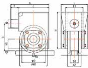
Unità di scorrimento folle
