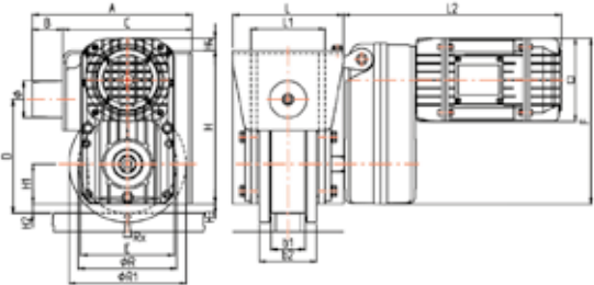
Unità di scorrimento motrice
