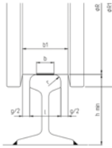
Binario in laminato quadro UNI 6013 - DIN 1013 Binario in laminato piatto UNI 6014 - DIN 1017 Binario tipo Burbak - DIN 536 Binario tipo Vignole - UNI 3141
