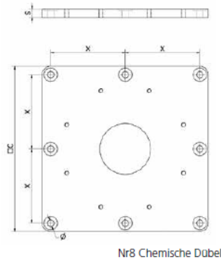
GEGENPLATTE T
