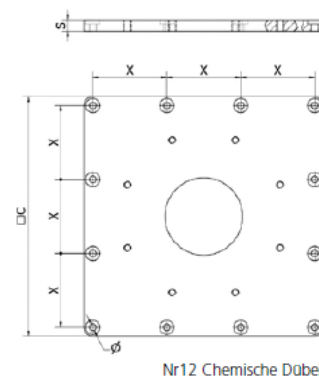
GEGENPLATTE U - V - Z1
