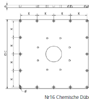
GEGENPLATTE Z2
