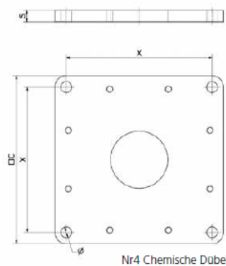
GEGENPLATTE R - S
