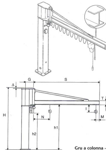
Gru a colonna - Rotazione 280°
