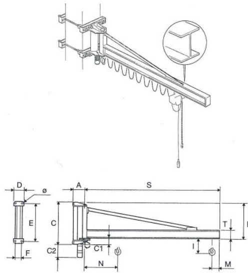
Gru a parete - Rotazione 290°
